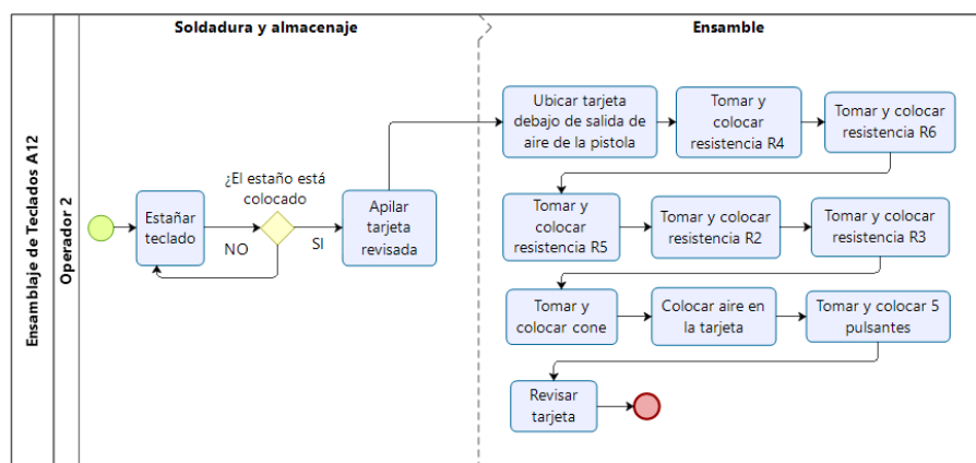
GRÁFICO 1. Diagrama de flujo de proceso de ensamblaje de teclados A12 Elaboración propia a partir de las fichas de levantamiento de procesos para la empresa de producción semiautomatizada de tarjetas electrónicas
