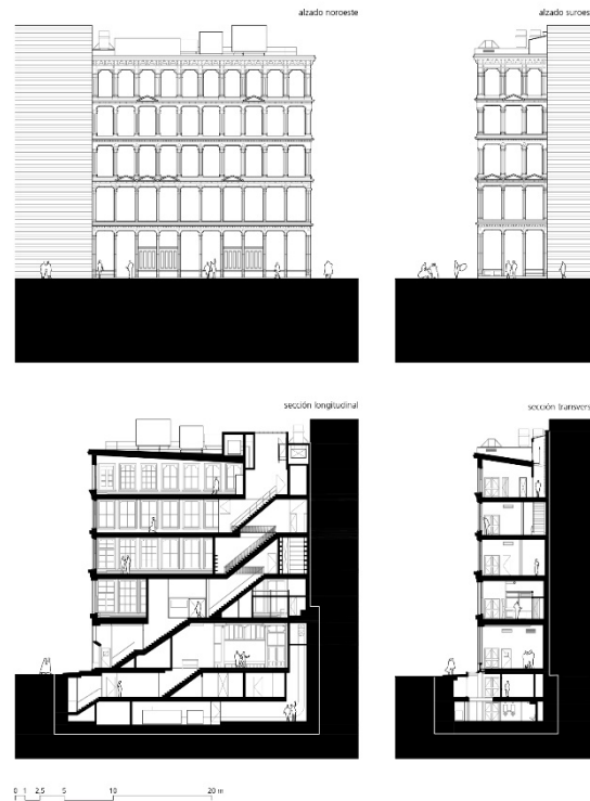
Figura 2. Plantas del edificio en el 101 Spring Street de la ciudad de Nueva York. Fuente: Elaboración propia.
