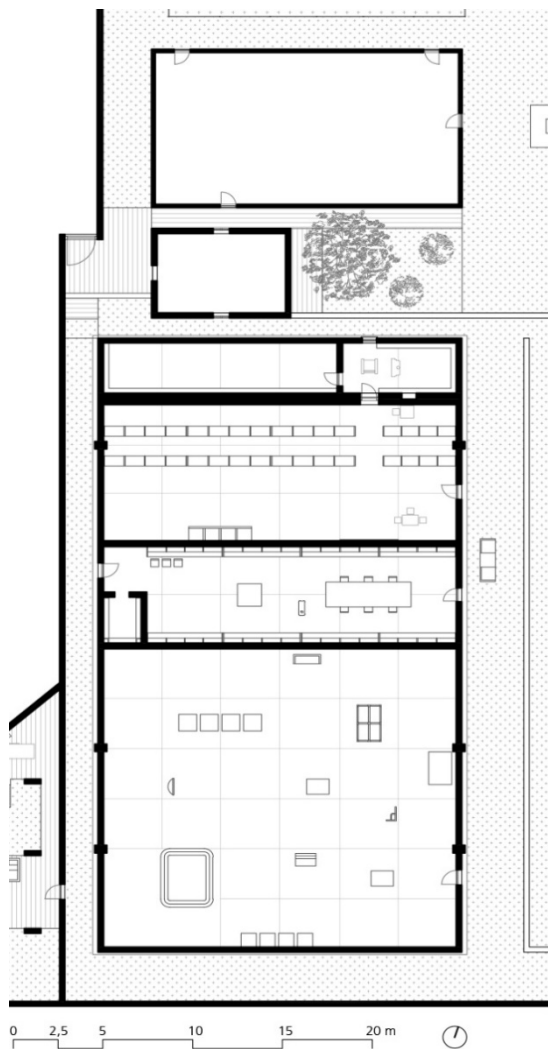
Figura 7. Planta de las construcciones de La Mansana de Chinati en Marfa, del lateral oeste. Fuente: Elaboración propia.
