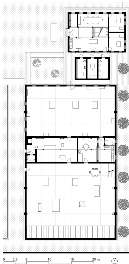
Figura 8. Planta de las construcciones de La Mansana de Chinati en Marfa, del lateral este. Fuente: Elaboración propia.
