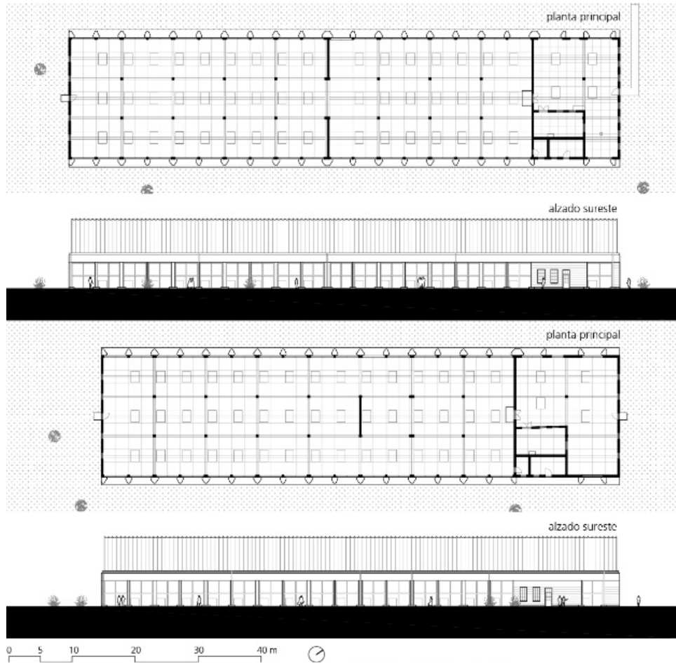
Figura 12. Plantas principales y alzados de los Artillery Sheds en Marfa. Fuente: Elaboración propia.
