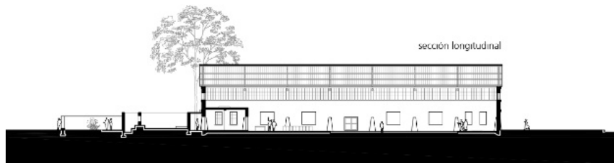
Figura 18. Planta principal, alzado y sección del Arena Building en Marfa. Fuente: Elaboración propia.
