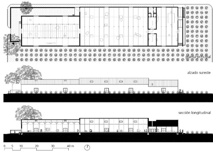
Figura 15. Planta principal, alzado y sección del Chamberlain Building en Marfa. Fuente: Elaboración propia.
