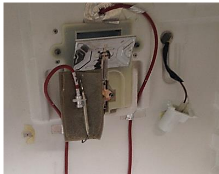
Figura 14. Montaje de termoresistores internos Fuente: Autores
